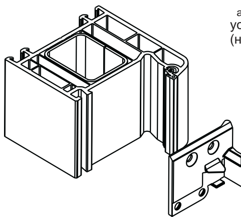
держатель для порога уплотнительная прокладка
