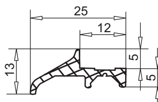
алюминиевый слезник 25/12 мм арт. № 104.171.001 алюминий с белым напылением арт. № 104.171.002 алюминий с коричневым напылением
