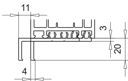
присоединительный профиль арт.№ 109.071 клипсовое соединение на раму
