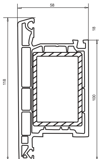
арт. № 105.124 дверная створка открывается наружу пленка с двух сторон усилитель арт. № 113.011.3
