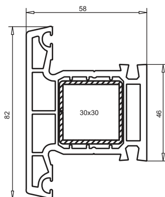
арт. № 102.103 пленка с двух сторон пленка с одной стороны усилитель арт. № 113.025 сварка только в соединении с рамой
