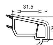
арт. №107.212 контур SOFTLINE
