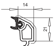
арт. №107.203 контур TOPLINE
