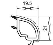
арт. №107.236 контур SWINGLINE
