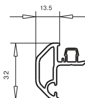
арт. № 109.560 упорная планка заглушка арт. №109.567
