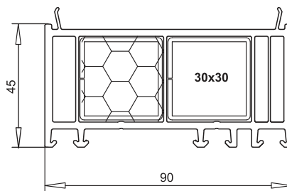
расширитель 45 мм арт.№ 114.206 усилитель арт.№ 113.025
