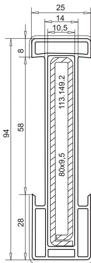
соединитель арт. № 116.044 стальная полоса арт. № 113.120.3 I_x=0,67 \text{ см}^4 , I_y=42,67 \text{ см}^4 усилитель арт. № 113.149.2 I_x=0,46 \text{ см}^4 , I_y=20,93 \text{ см}^4
