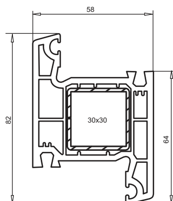
арт. № 102.130 переходной профиль пленка с двух сторон усилитель арт. № 113.025 сварка только с 102.103!
