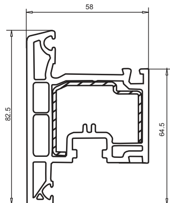
арт. № 103.213 усилитель арт. № 113.229
