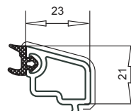
арт. №107.210 контур SOFTLINE
