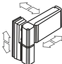
арт. № 140.318 петля VEKA для входной двери из двух частей, для створки весом до 120 кг регулируется в 3 плоскостях, установка с обеих сторон цвет: белый / Euras 15 (коричневый) шаблон арт. № 146.011.7
