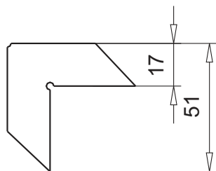
ПВХ - уголок для 109.187/ 188 Цвет: белый арт.№ 109.189
