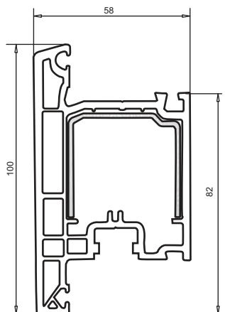
арт. № 103.219 дверная створка открывается наружу пленка с двух сторон усилитель арт. № 113.049.2 усилитель арт. № 113.147.2
