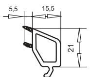
арт. №107.217 контур SOFTLINE
