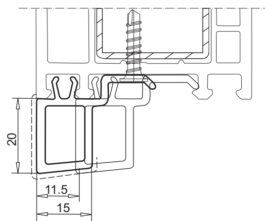
профиль для присоединения отлива арт. № 110.048
