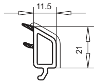
арт. №107.218 контур SOFTLINE
