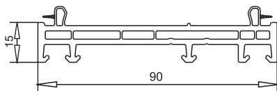
расширитель 15 мм арт.№ 114.208
