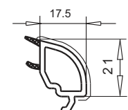
арт. №107.237 контур SWINGLINE
