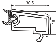
штапик арт. № 107.569
