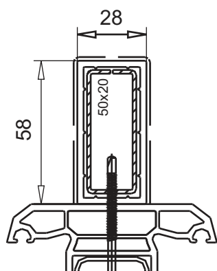
внешний усилитель 28x58мм арт.№ 109.082 усилитель арт.№ 113.047 I_x=1,41\text{см}^4 , I_y=6,21\text{см}^4
