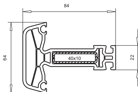
арт. № 102.243 створочная перекладка пленка с двух сторон пленка с одной стороны усилитель арт. №113.028
