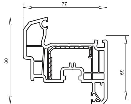
арт. № 103.239 пленка с двух сторон пленка с одной стороны усилитель арт. №113.292 усилитель арт. №113.294 усилитель арт. №113.295
