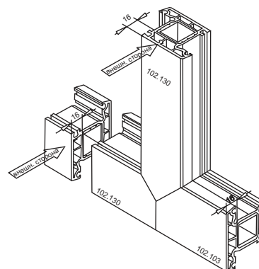
арт. № 102.130 переходной профиль пленка с двух сторон усилитель арт. № 113.025 сварка только с 102.103!
