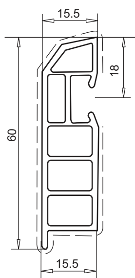
маскирующий профиль
