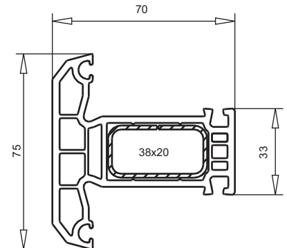
арт. № 102.201 пленка с двух сторон пленка с одной стороны усилитель арт. №113.272
