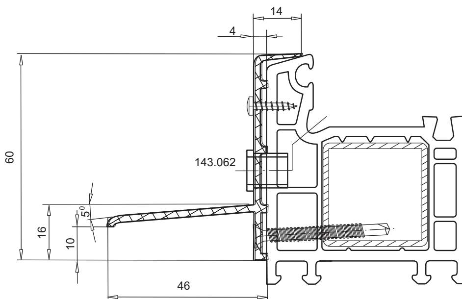
алюмин. порожек арт. № 104.046 цвет: алюмин., E6/EV1 Euras15
