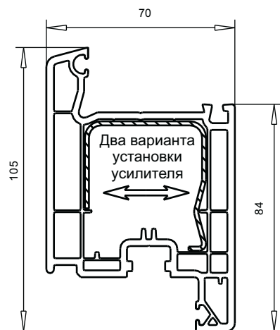
арт. № 103.241 пленка с двух сторон пленка с одной стороны усилитель арт. № 113.270 алюмин. арт. № 115.003
