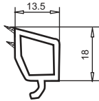
штапик арт. № 107.213 толщина стеклопакета 24+24,5 мм
