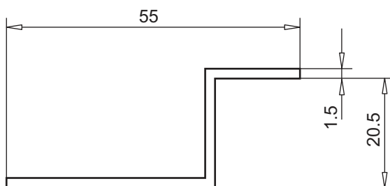
Z-образный профиль арт. № 117.834
