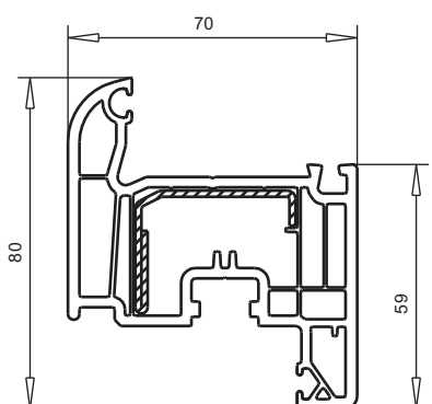
арт. № 103.235 пленка с двух сторон пленка с одной стороны усилитель арт. №113.292 усилитель арт. №113.294 усилитель арт. №113.295
