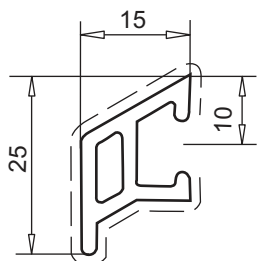
защитная планка
