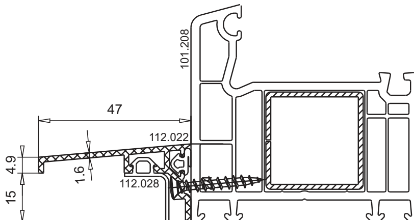
защитный порожек арт.№ 104.421 цвет: алюминий, белый, черный
