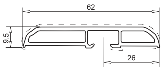
маскирующий профиль
