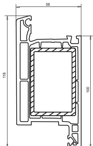
арт. № 105.123 дверная створка усилитель пленка с двух сторон пленка с одной стороны арт. № 113.011.3
