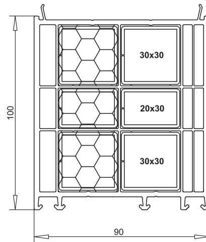
расширитель 100 мм арт.№ 114.207 усилитель арт. № 113.025 усилитель арт. № 113.019
