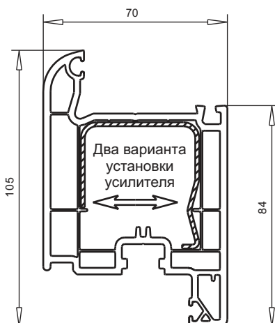
арт. № 103.273 пленка с двух сторон пленка с одной стороны усилитель арт. №113.270 алю.усилитель арт. №115.003
