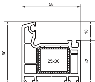
арт. № 101.287 усилитель арт. № 113.002 усилитель арт. № 113.060
