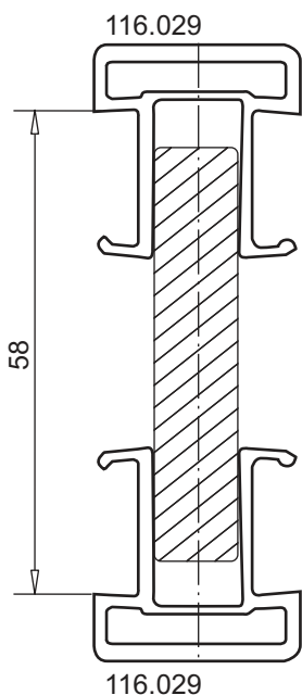
накладка для полосы арт. № 116.029 / 2x усилитель арт. № 113.013.3 I_x=0,42 \text{ см}^4 , I_y=10,42 \text{ см}^4
