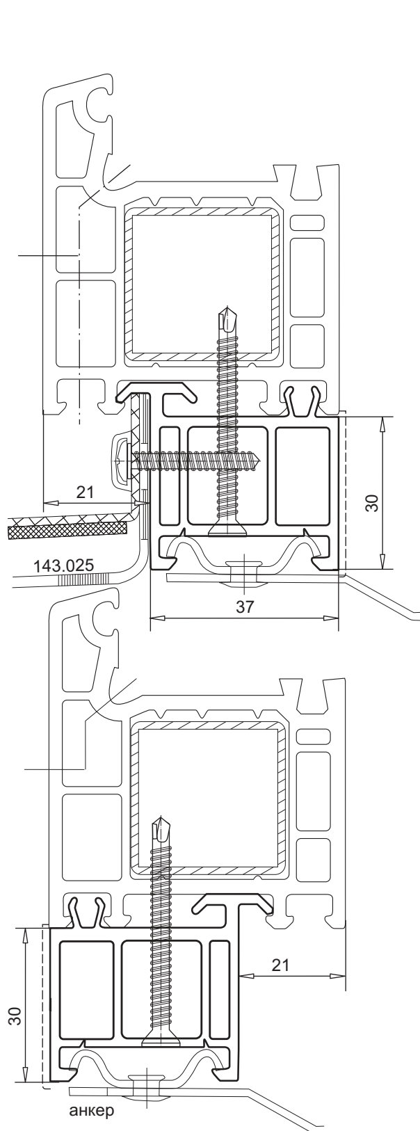
профиль для присоединения балконной двери 30 мм арт. № 109.304
