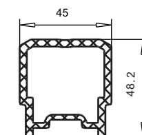
усилитель арт. № 113.295 (для нестандарт. конструкций)
