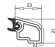
арт. №107.200 контур TOPLINE
