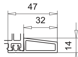
облицовочный профиль арт.№ 109.231 клипсовое соединение на раму
