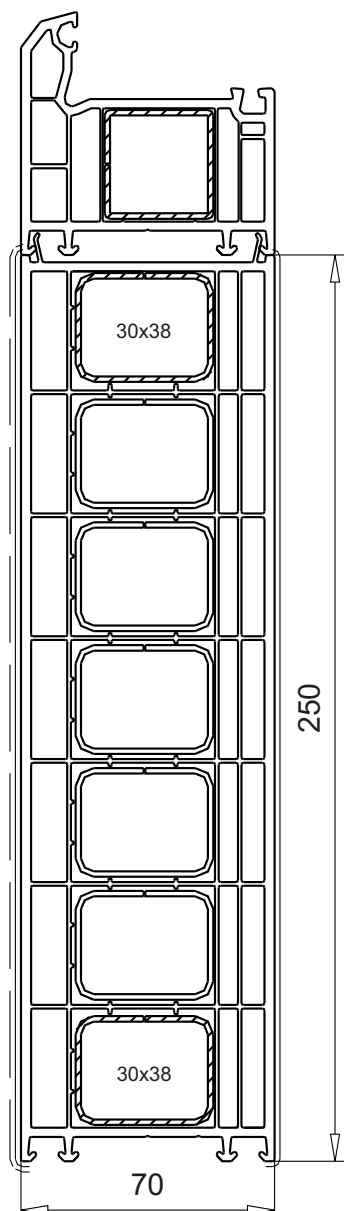
расширитель 250мм арт.№ 114.205 усилитель арт.№ 113.271 усилитель арт.№ 113.271.4
