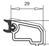
арт. №107.206 контур TOPLINE
