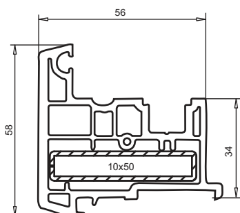
арт. № 102.196 штульп пленка с двух сторон пленка с одной стороны усилитель арт. № 113.013 стальная полоса арт. № 113.013.3 размер штульпа: высота створки-72 мм
