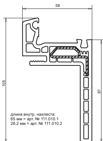
арт. № 111.010 усилитель арт. № 113.181
