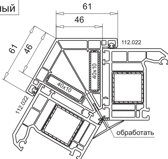
угловой соединитель 120° арт.№ 116.016 усилитель арт.№ 113.028 lx=0,23см4, ly=2,38см4
