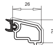
арт. №107.207 контур TOPLINE
