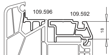
вставка арт. № 109.592 фальцевый вкладыш арт. № 109.596 Цвет: красный
