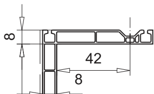
облицовочный профиль 185мм арт.№ 109.186
