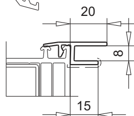
профиль с пазом арт.№ 109.286
