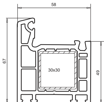
арт. № 101.086 пленка с двух сторон пленка с одной стороны усилитель арт. № 113.025
