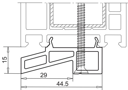
профиль для присоединения отлива арт. № 110.019
