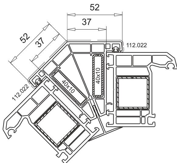
угловой соединитель 135° арт. № 116.015 усилитель арт.№ 113.028 lx=0,23см4, ly=2,38см4
