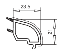
арт. №107.235 контур SWINGLINE
