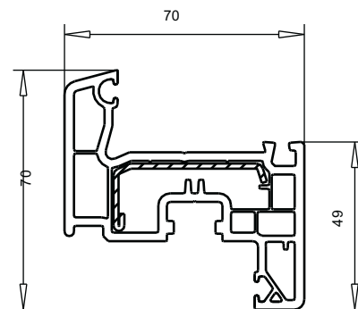
арт. № 103.229 пленка с двух сторон пленка с одной стороны усилитель арт. № 113.269
