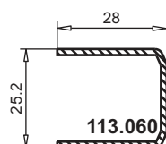
арт. № 101.287 усилитель арт. № 113.002 усилитель арт. № 113.060
