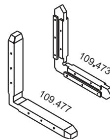
уголок для 111.031/111.032 Цвет: белый арт.№ 109.473 для плеча 50мм арт.№ 109.477 для плеча 70 / 156мм
