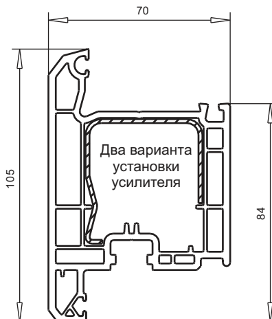
арт. № 103.203 наружное открывание пленка с двух сторон усилитель арт. №113.270 алюмин.усилитель арт.№115.003 (только для белых профилей)
