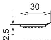
маскирующий профиль 30мм арт.№ 109.439.3 с резинкой, белый с клеящейся лентой 19x1мм, черный
