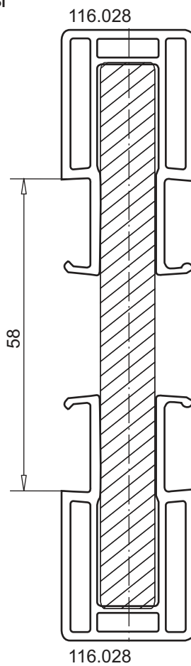
накладка для полосы арт. № 116.028 / 029 усилитель арт. № 113.120.3 I_x=0,67 \text{ см}^4 , I_y=42,67 \text{ см}^4
