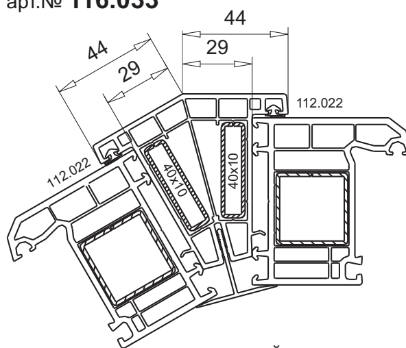
угловой соединитель 150°
