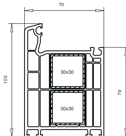
арт. № 101.215 пленка с двух сторон пленка с одной стороны усилитель арт. № 113.025
