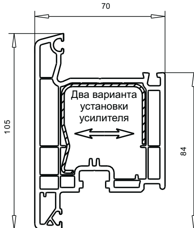
арт. № 103.242 наружное открывание пленка с двух сторон усилитель арт. № 113.270 алюмин. арт. № 115.003
