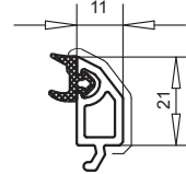
арт. №107.204 контур TOPLINE
