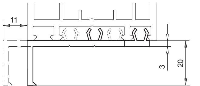
4 присоединительный профиль арт. № 109.071
