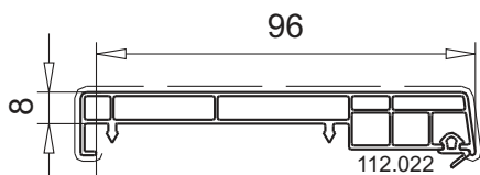
облицовочный профиль арт.№ 109.188 клипсовое соединение
