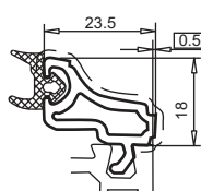
штапик арт. № 107.555
