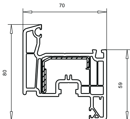
арт. № 103.232 пленка с двух сторон пленка с одной стороны усилитель арт. № 113.292 (белый) усилитель арт. № 113.294 (цветной)
