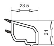
арт. №107.244 контур TOPLINE
