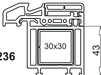
арт. № 109.445 усилитель 113.025 (на выбор)
