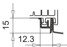
алюм. соединительный профиль арт.№ 104.228 клипсовое соединение на раму
