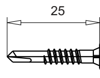
шуруп 4,2 x 25мм с самонарезающей головкой арт.№ 141.007.025
