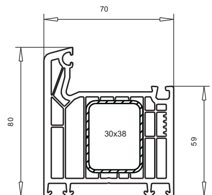
арт. № 101.285 SOFTLINE XXL усилитель арт. № 113.271 усилитель арт. № 113.302
