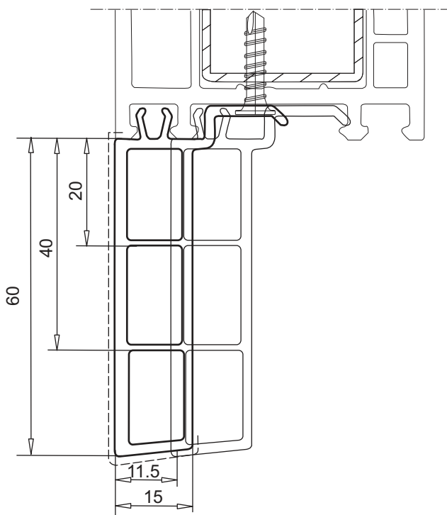
профиль для присоединения отлива арт. № 110.101
