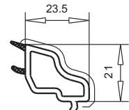
арт. №107.226 контур SOFTLINE
