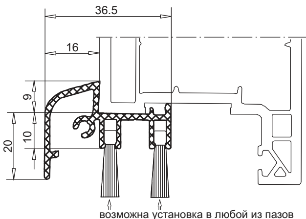
алюминиевая защитная планка
