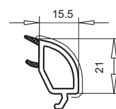
арт. №107.238 контур SWINGLINE
