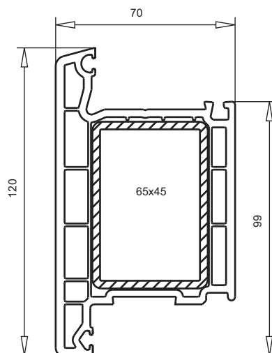
арт. № 105.233 дверная створка наружного открывания пленка с двух сторон усилитель арт. № 113.286.3 алюмин.усилитель арт. № 115.200
