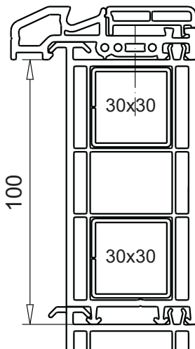
арт. № 109.437 усилитель арт.№ 113.025 (на выбор)
