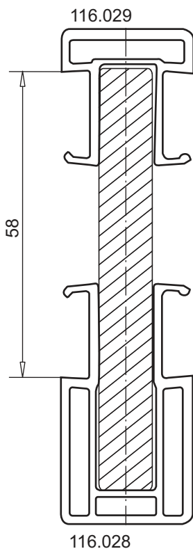
накладка для полосы арт. № 116.028 / 029 усилитель арт. № 113.120.3 I_x=0,67 \text{ см}^4 , I_y=42,67 \text{ см}^4
