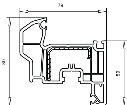
арт. № 103.238 пленка с двух сторон пленка с одной стороны усилитель арт. № 113.292 (белый) усилитель арт. № 113.294 (цветной) спец.усилитель арт. № 113.295
