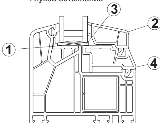
Глухое остекление
