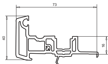
арт. № 102.197 штульп пленка с двух сторон пленка с одной стороны размер штульпа: высота створки-72 мм
