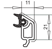
арт. №107.220 контур SOFTLINE
