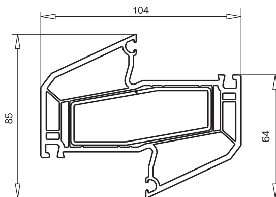
арт. № 102.231 переходной профиль усилитель арт. №113.331/113.343.2
