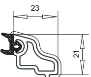
арт. №107.211 контур SOFTLINE
