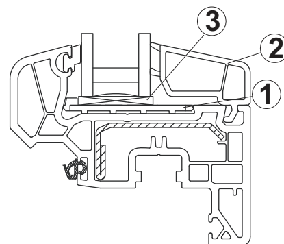
Остекление створки
