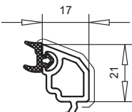
арт. №107.202 контур TOPLINE
