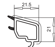
арт. №107.224 контур SOFTLINE
