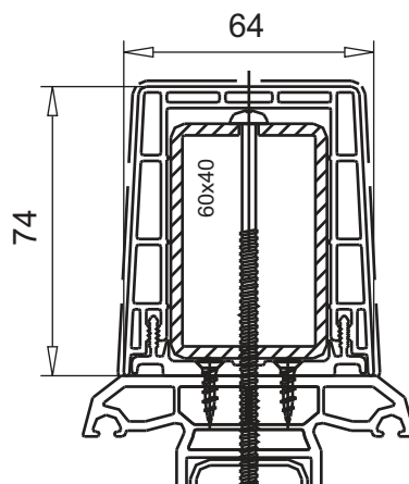
внешний усилитель 64x74мм арт.№ 114.031 усилитель арт.№113.011.2 I_x=10,23\text{см}^4 , I_y=19,31\text{см}^4 усилитель арт.№113.011.3 I_x=14,32\text{см}^4 , I_y=27,39\text{см}^4
