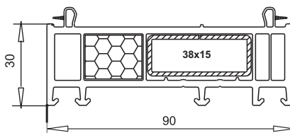
расширитель 30 мм арт.№ 114.209 усилитель арт.№ 113.073
