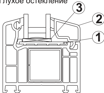
Глухое остекление
