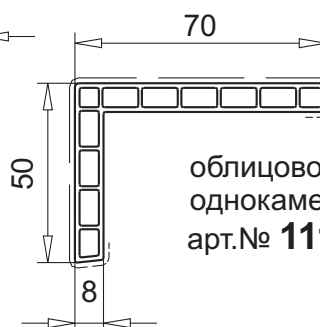
облицовочный однокамерный профиль арт.№ 111.032
