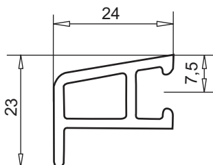
маскирующий профиль
