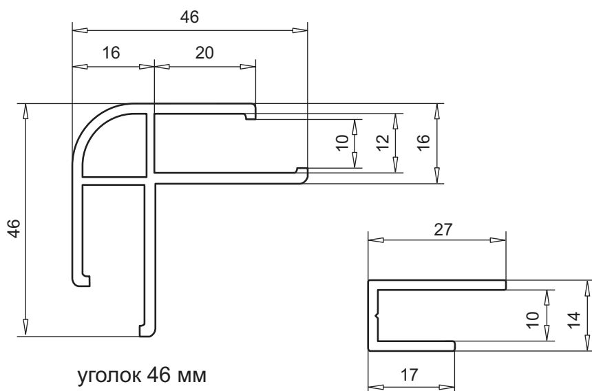
П-образный профиль арт. № 109.254
