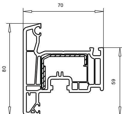
арт. № 103.228 наружное открывание пленка с двух сторон усилитель арт. № 113.292 (белый) усилитель арт. № 113.294 (цветной) спец.усилитель арт. № 113.295
